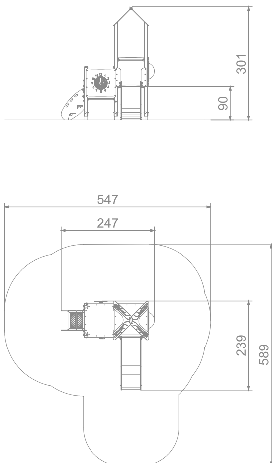
SKALA 1:100
